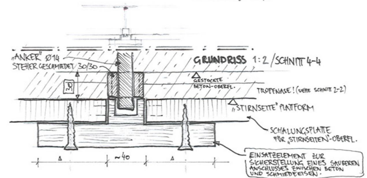
GRUNDRISS 1:10
